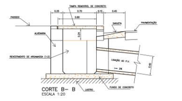
DETALHAMENTO BOCA DE LOBO DUPLA SEM ESCALA
