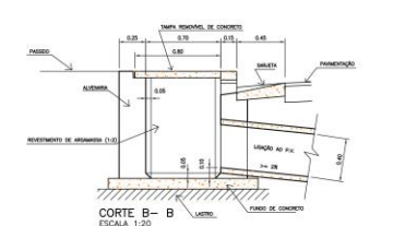
DETALHAMENTO BOCA DE LOBO SIMPLES SEM ESCALA
